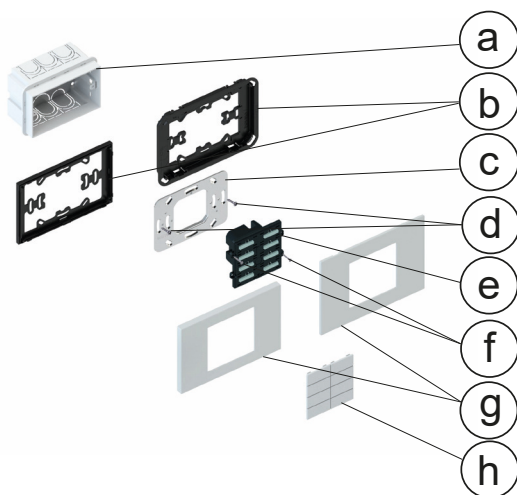
Montaggio per scatola rettangolare
