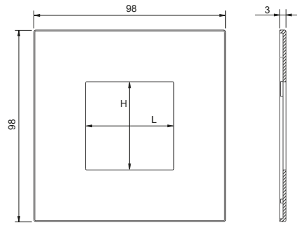
Placca EK-SQT... (4 tasti) Placca EK-SQS... (8 tasti) serie Surface
