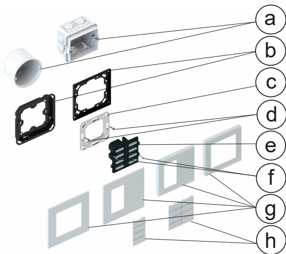
Montaggio per scatola quadrata o rotonda
