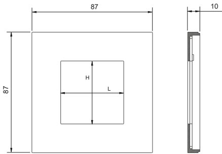
Placca EK-DQT... (4 tasti) Placca EK-DQS... (8 tasti) serie Deep
